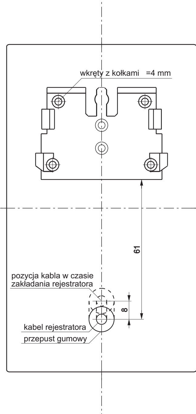
Szablon do trasowania otworów obudowy BB01
